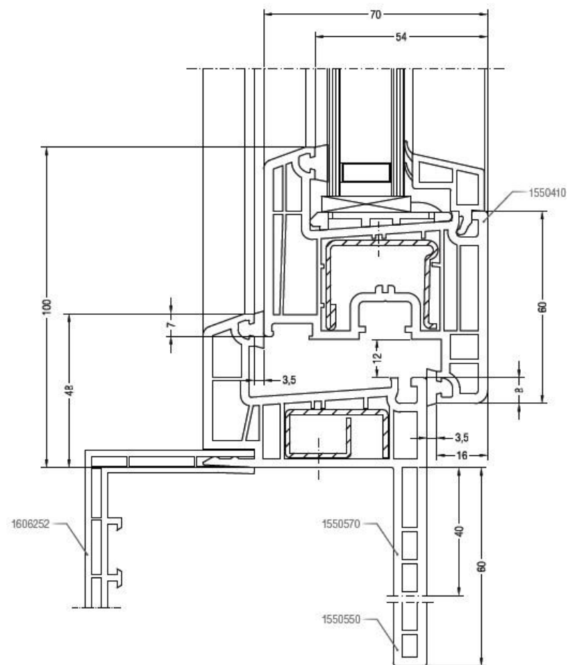
Sezione nodo Brillant 70 telaio Z ( aletta da 60 mm ) – anta dritta
