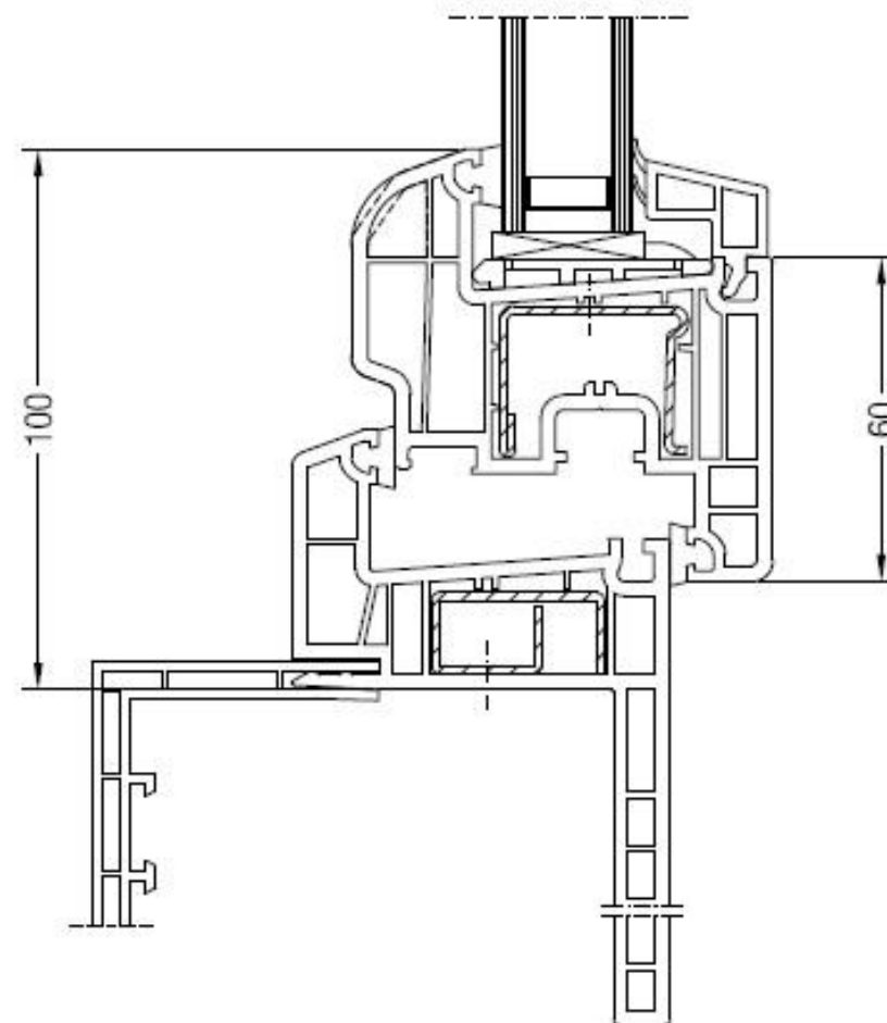
Sezione nodo Brillant 70 telaio Z ( aletta da 60 mm ) – anta arrotondata
